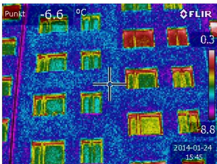
Temperatura powierzchni ocieplenia etics na elewacji północno-zachodniej
